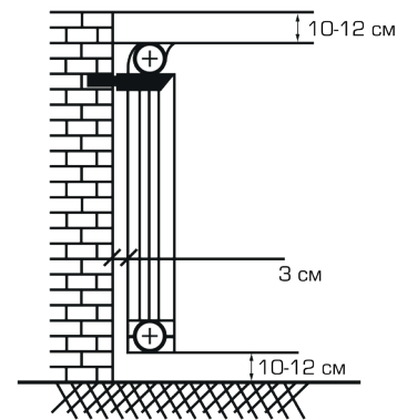
Рис. 2. Правила установки радиатора
